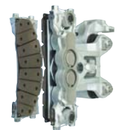
新幹線用ディスクブレーキ
